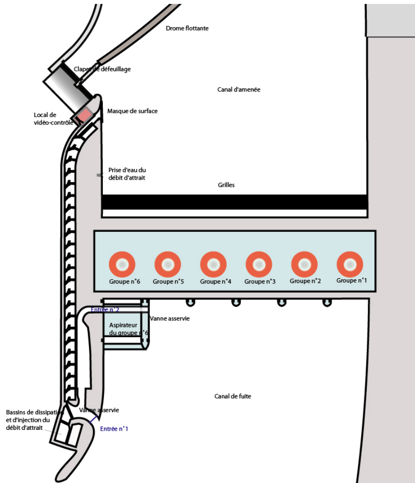
Schéma de l'usine hydroélectrique de Mauzac
