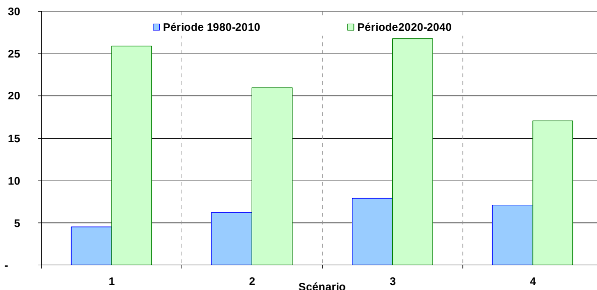
Nombre moyen de jours où la température de l'estuaire limite la production pour les quatre scénarii pour les périodes 1980-2010 et 2020-2040
