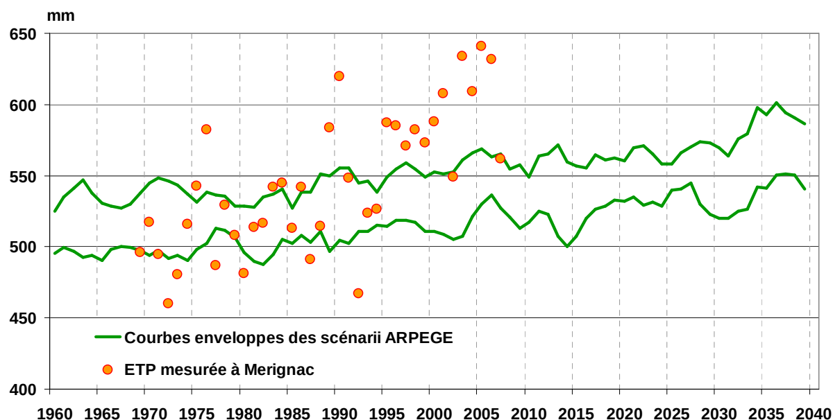
Comparaison de l'ETP estivale mesuré à Mérignac et celles simulées à l'aide du modèle Cerfacs
