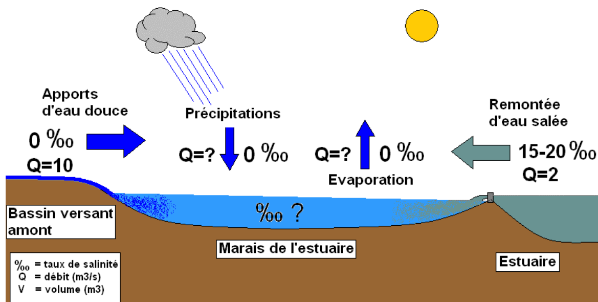
Schématisation globale montrant la potentialité saline du marais
