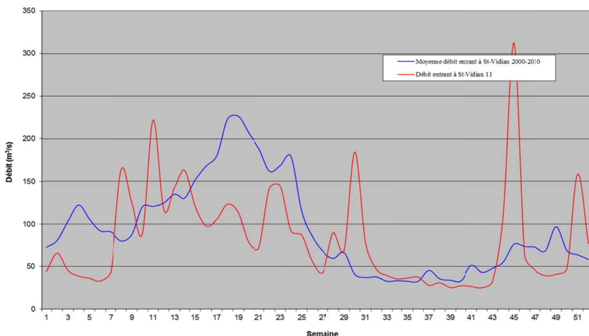
Figure 7 : Evolution du débit de la Garonne en amont de Carbone (St Vidian) entre le 1/01/11 et le 31/12/11. Comparaison avec la moyenne de 2000 à 2010
