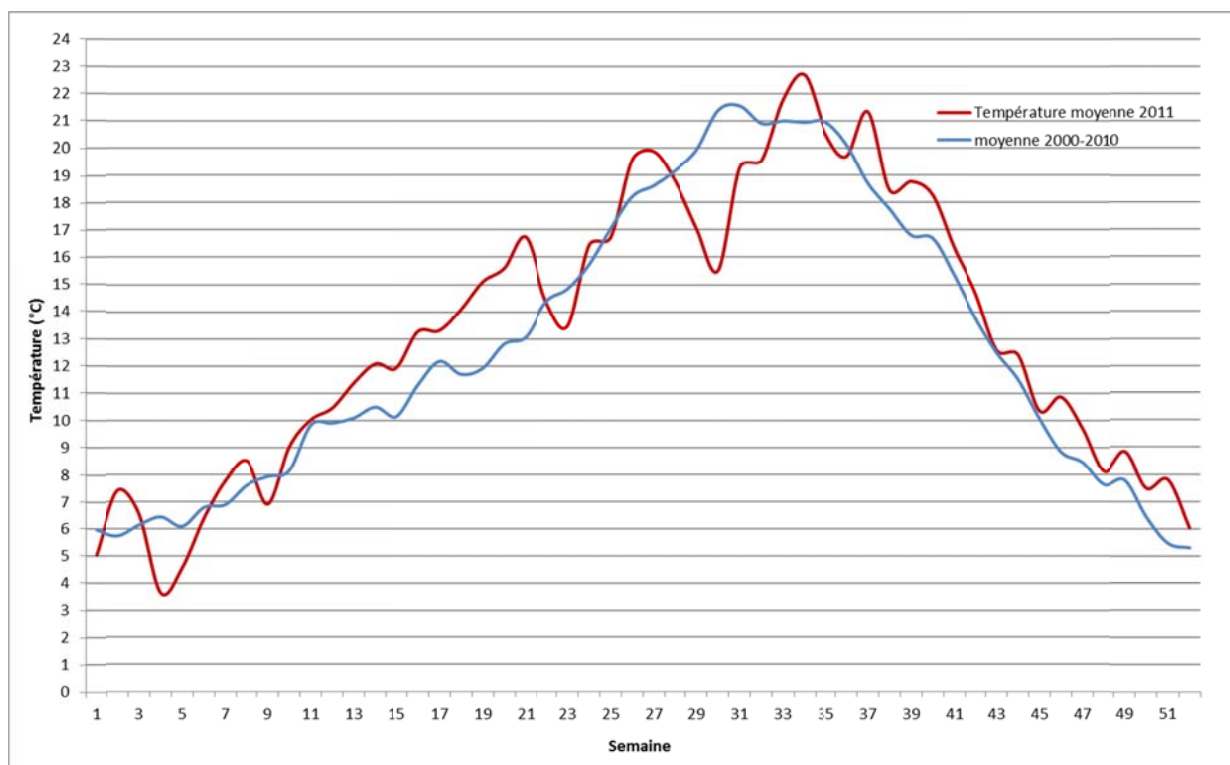
Figure 8 : Evolution de la température moyenne de la Garonne à Carbonne entre le 01/01/11 et le 31/12/11. Comparaison avec la moyenne de 2000 à 2010
