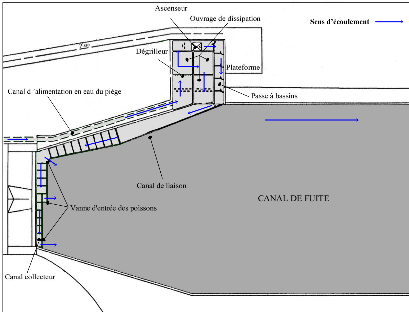
Figure 4 : Sens d'écoulement de l'eau dans la station de piégeage de Carbone
