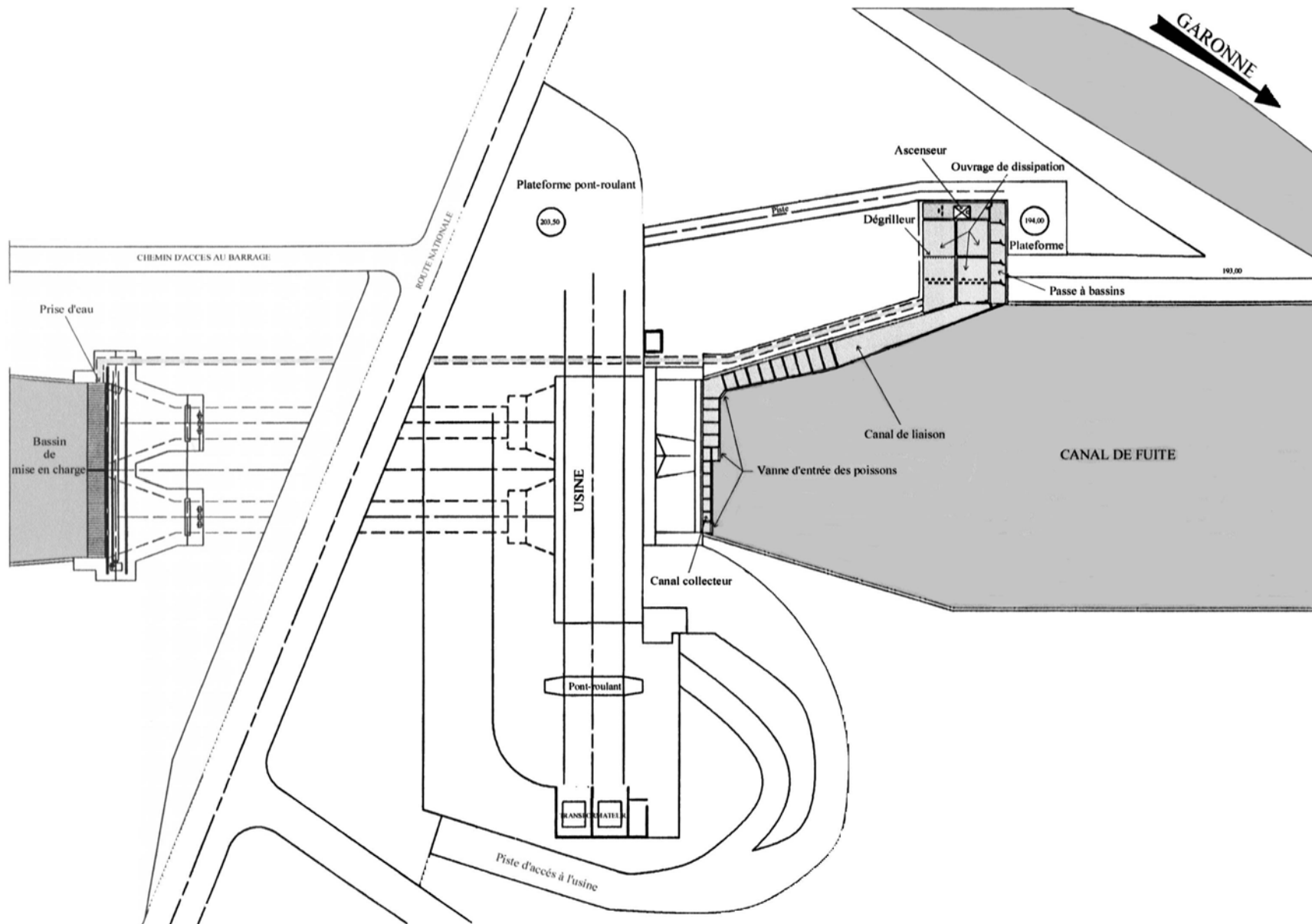
Figure 3 : Situation de la station de piégeage au niveau de l'aménagement hydroélectrique EDF de Carbonne
