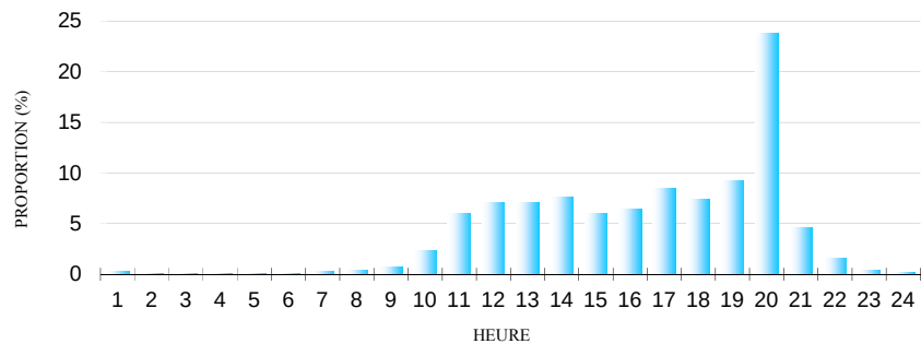
ACTIVITE Horaire DES BREMES AU BAZACLE EN 2016
