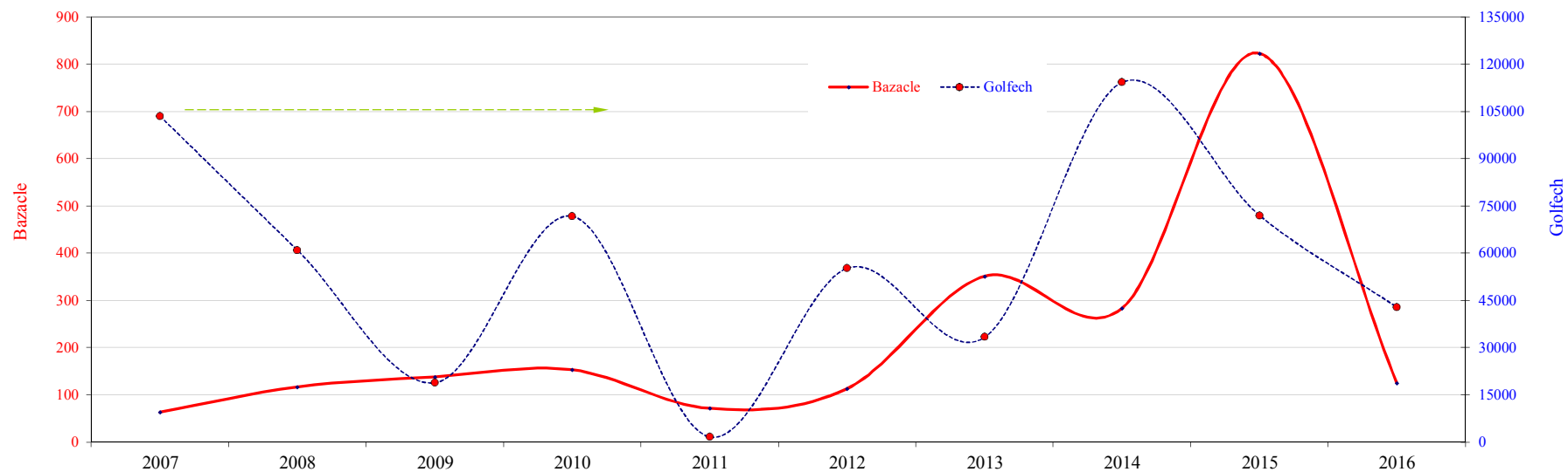
FIGURE 16 : EVOLUTION COMPAREE DES EFFECTIFS D'ANGUILLE AU BAZACLE ET A GOLFECH
