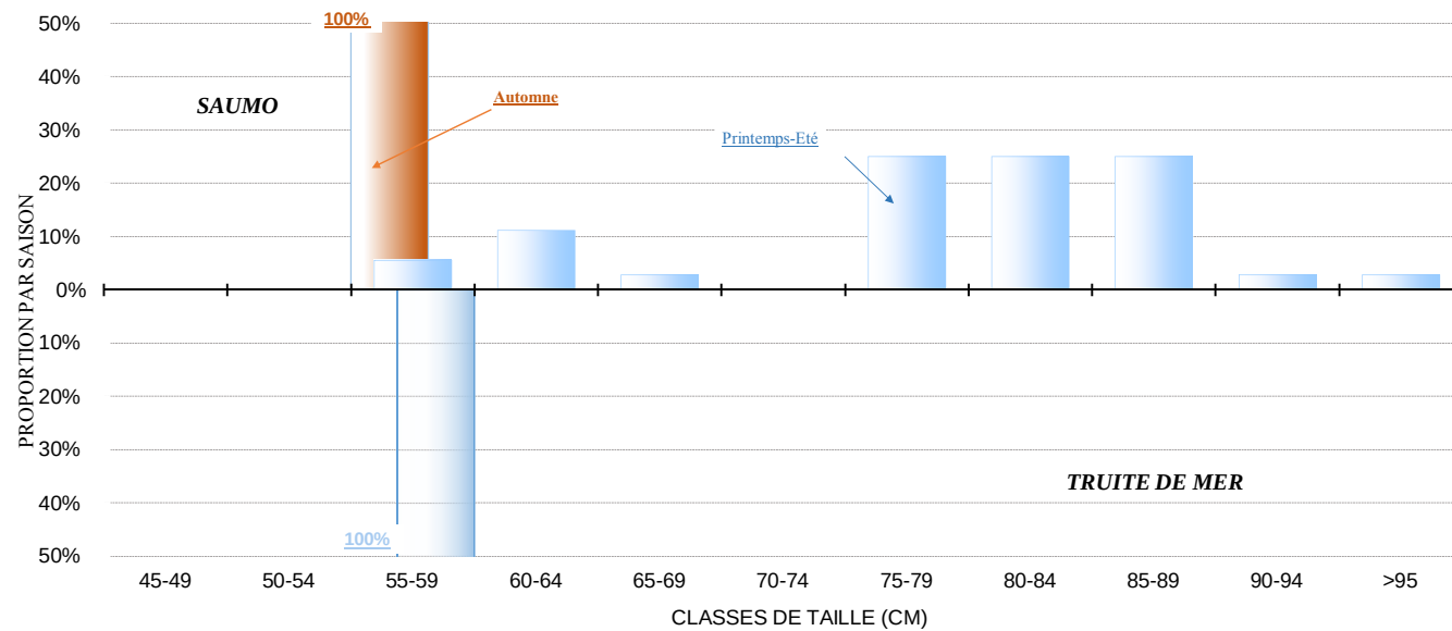
FIGURE 10 : HISTOGRAMMES COMPARES DES TAILLES DE SALMONIDES AU BAZACLE EN 2016
