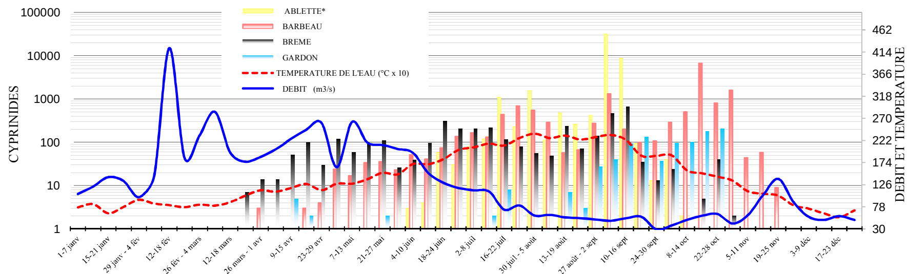
FIGURE 11 : MIGRATIONS DES CYPRINIDES ET CONDITIONS ENVIRONNEMENTALES AU BAZACLE EN 2016
