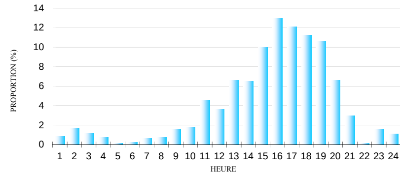
ACTIVITE Horaire DES GARDONS AU BAZACLE EN 2016
