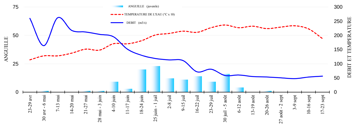
FIGURE 8 : HISTOGRAMME DES TAILLES DES ANGUILES AU BAZACLE EN 2016
