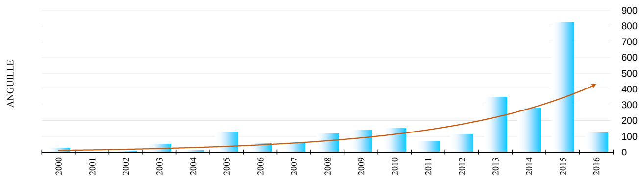
FIGURE 6 : MIGRATION DES ANGUILES AU BAZACLE DEPUIS 2000
