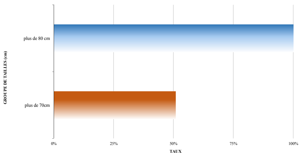
FIGURE 15 : TAUX DE TRANSFERT DES SAUMONS ENTRE GOLFECH ET LE BAZACLE SELON LE GROUPE DE TAILLES EN 2016
