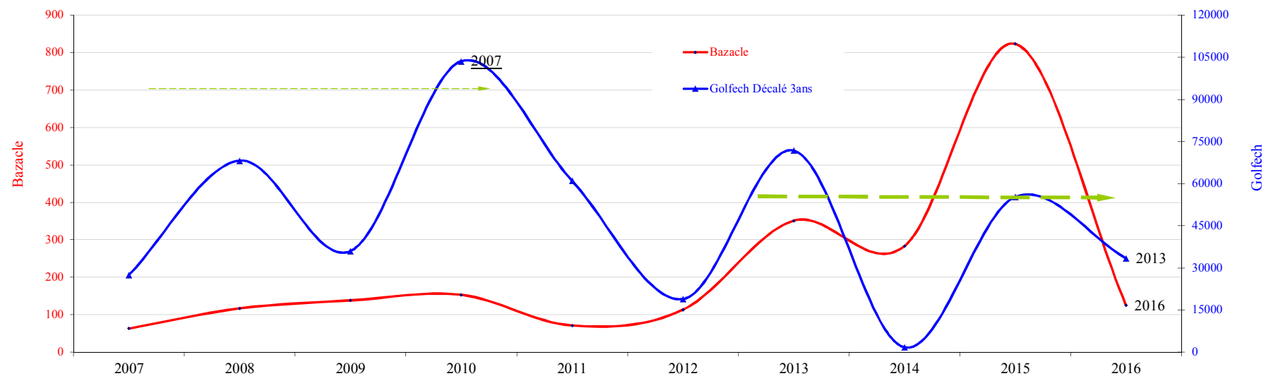
FIGURE 16.1 : EVOLUTION COMPAREE DES EFFECTIFS D'ANGUILLE AU BAZACLE ET A GOLFECH : ARRIVEE DECALEE DE 3 ANS
