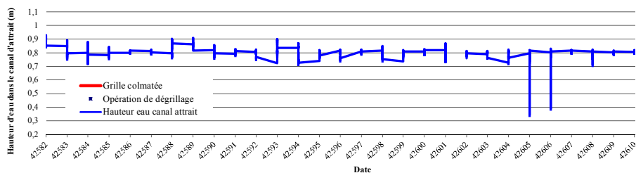
Evolution du colmatage de la grille amont de l'attrait au Bazacle au mois de septembre 2016
