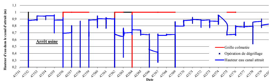
Evolution du colmatage de la grille amont de l'attrait au Bazacle au mois de août 2016
