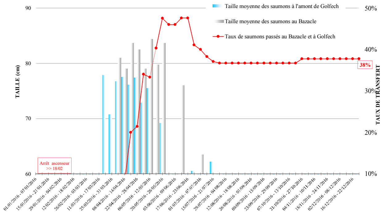
FIGURE 14 : EVOLUTION PAR SEMAINE DU TAUX DE TRANSFERT DES SAUMONS ENTRE GOLFECH ET LE BAZACLE, ET DE LA TAILLE MOYENNE EN 2016
