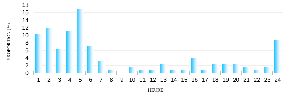
ACTIVITE Horaire DES ANGUILES AU BAZACLE EN 2016
