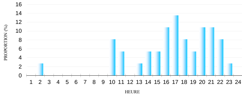
ACTIVITE Horaire DES SAUMONS AU BAZACLE EN 2016
