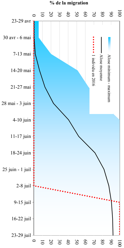
MIGRATIONS CUMULEES DES ALOSES AU BAZACLE DEPUIS 1989
