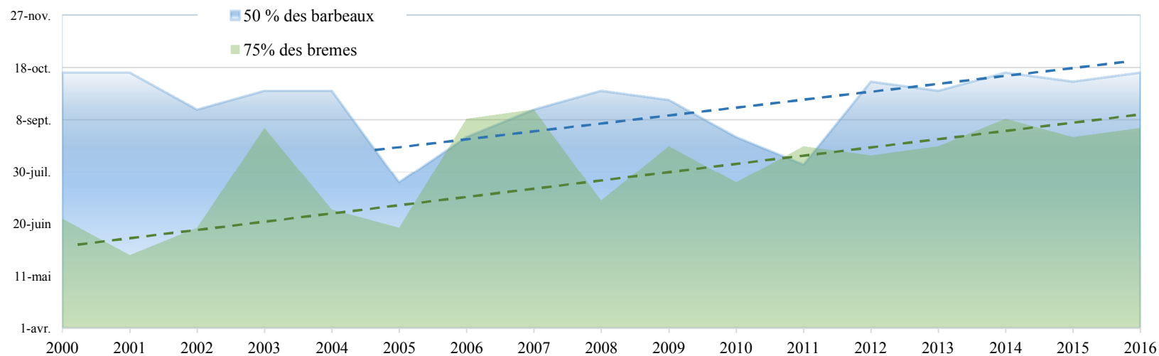
Figure 11.1 : Evolution de la date des passages des migrations de barbeaux et de bremes au Bazacle
