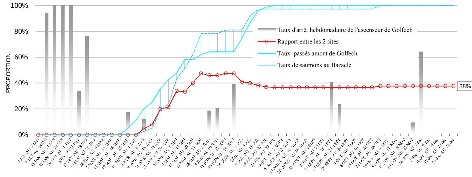
FIGURE 13 : COMPARAISON DES PASSAGES CUMULES DES SAUMONS PASSES A L'AMONT DE GOLFECH ET AU BAZACLE EN 2016
