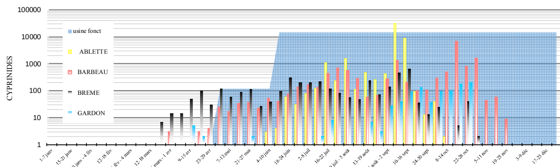
FIGURE V.13 : MIGRATIONS DES CYPRINIDES ET USINE AU BAZACLE EN 2016
