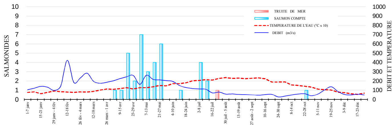
FIGURE 9 : MIGRATIONS DES SALMONIDES ET CONDITIONS ENVIRONNEMENTALES AU BAZACLE EN 2016
