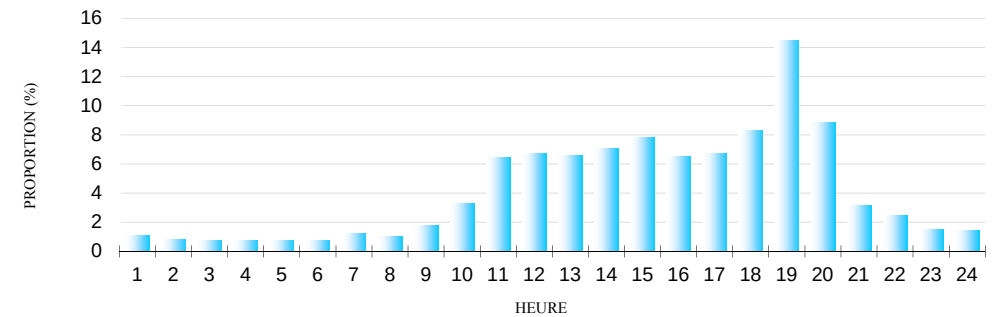
ACTIVITE Horaire DES BARBEAUX AU BAZACLE EN 2016
