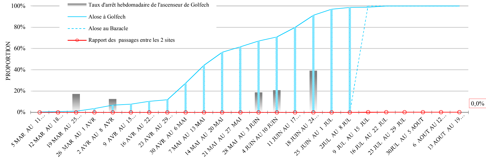
FIGURE 12 : COMPARAISON DES PASSAGES CUMULES D'ALLOSES A GOLFECH ET AU BAZACLE EN 2016
