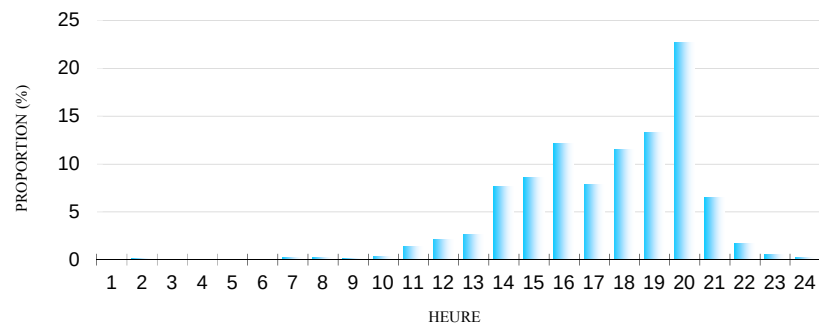
ACTIVITE Horaire DES ABLETTES AU BAZACLE EN 2016
