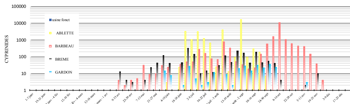
FIGURE V.12 : MIGRATIONS DES CYPRINIDES ET USINE AU BAZACLE EN 2015
