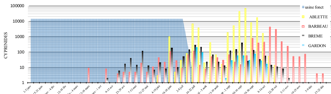
FIGURE V.11 : MIGRATIONS DES CYPRINIDES ET FONCTIONNEMENT USINE AU BAZACLE EN 2014
