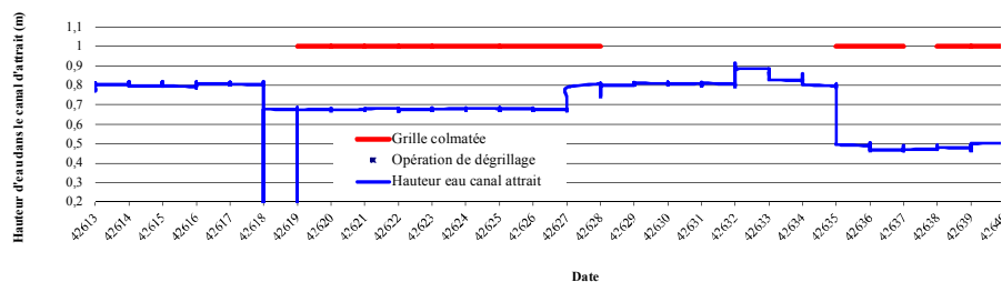
Evolution du colmatage de la grille amont de l'attrait au Bazacle au mois de octobre 2016
