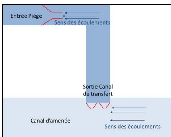
Figure 63 : Schéma représentant le sens des écoulements au droit de la grille anti retour et du piège au niveau du canal de transfert du dispositif de franchissement de Golfech.
