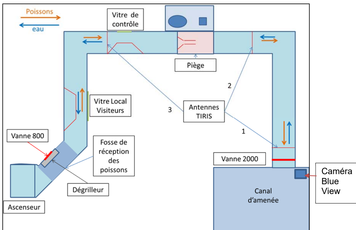
Figure 56 Schéma du canal de transfert de l'ascenseur à poissons de Golfech.
