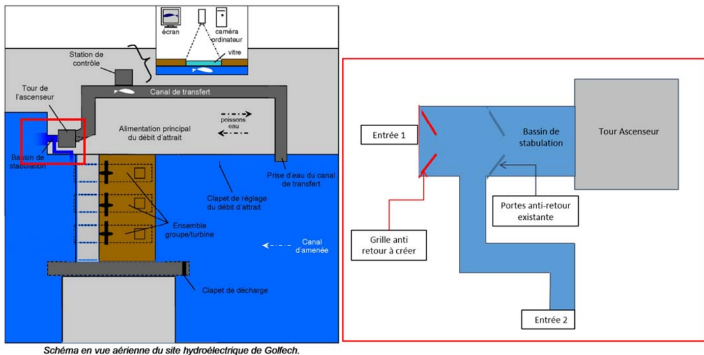
Figure 7 : Schéma de principe d'une grille anti retour au niveau de l'entrée 1 de l'ascenseur à poissons de Golfech
