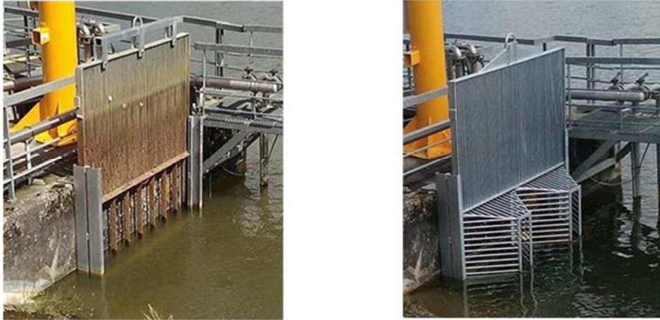
Figure 57 : Photo de l'ancienne grille située à l'amont du canal de transfert (gauche) et nouvelle grille « anti-retour » mise en place sur le site de Golfech en amont du canal de transfert en 2017.
