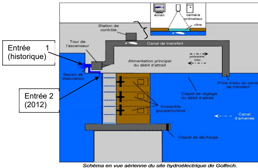
Figure 2 : Schéma en vue aérienne du site hydroélectrique de Golfech et de la station de contrôle
