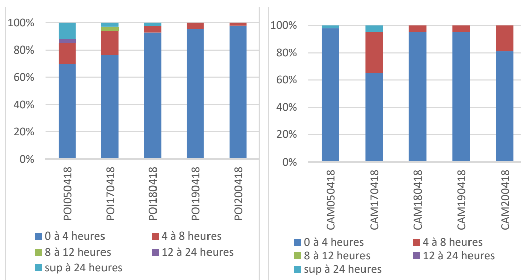
Figure 18 : Répartition dans le temps des recaptures de smolts marqués pour chaque lot lâché dans les canaux de Pointis (à gauche) et Camon (à droite)
