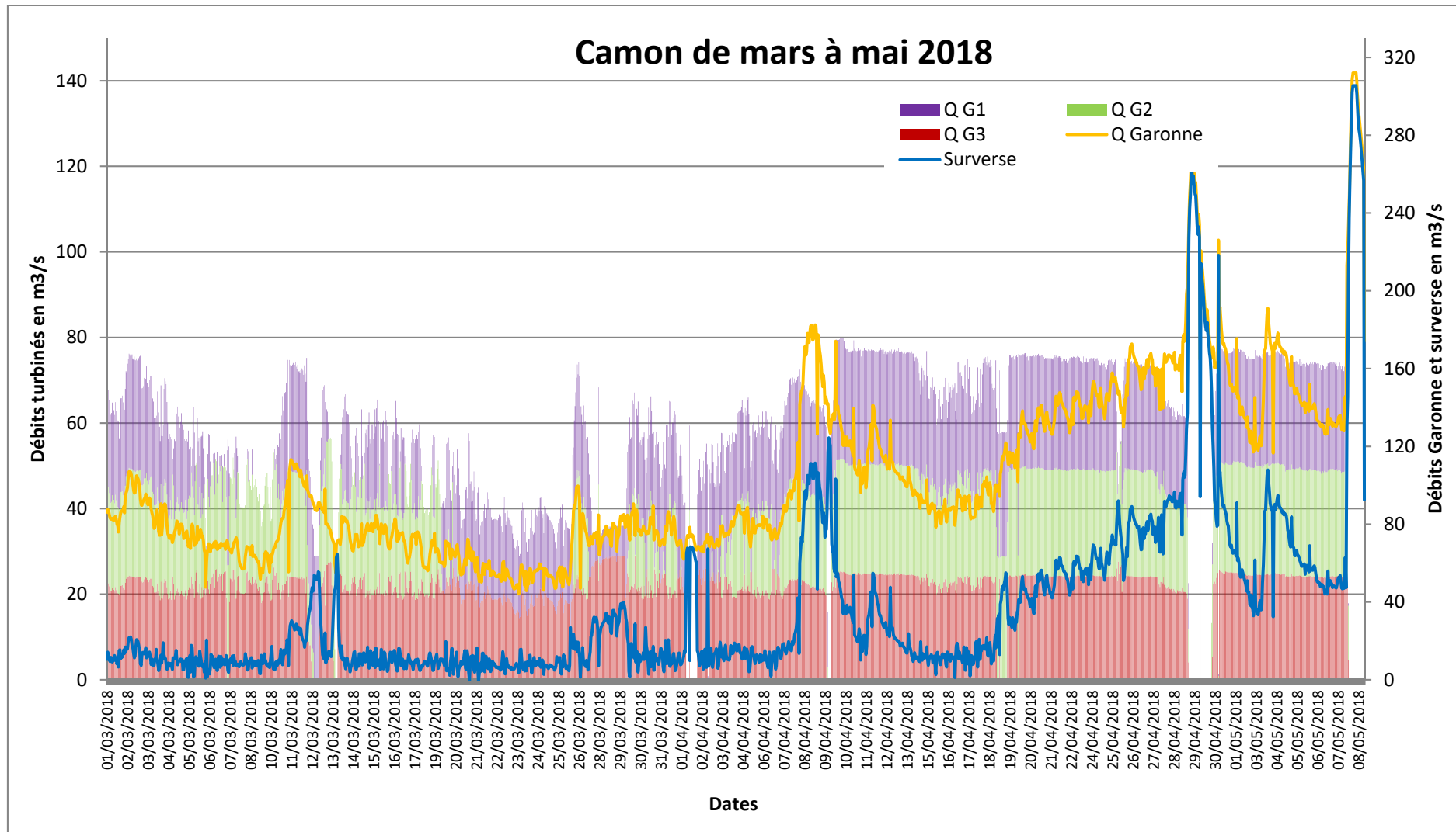
Figure 4 : Fonctionnement des groupes de l'usine de Camon et débit de la Garonne durant la campagne 2018 (débit en m³/s)
