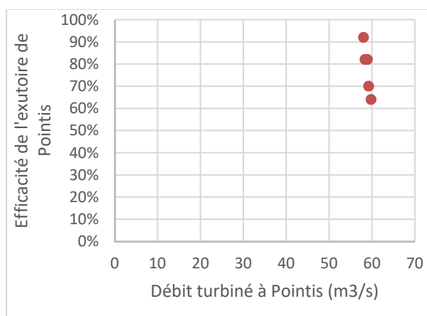
Figure 19 : Résultats d'efficacité des exutoires de Pointis pour chaque lot de smolts marqués en fonction des débits turbinés et des groupes en fonctionnement à l'usine.
