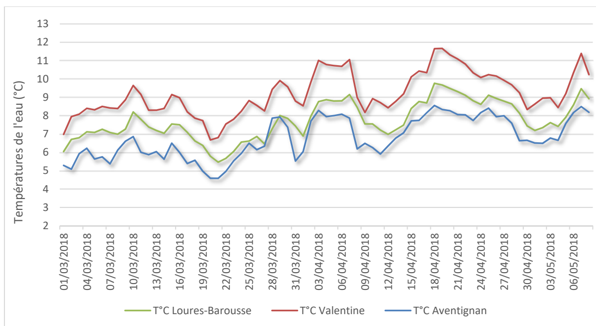
Figure 2 : Températures moyennes journalières (en °C) relevées sur la Garonne à Loures-Barousse et Valentine et sur la Neste à Aventignan pendant la période d'étude
