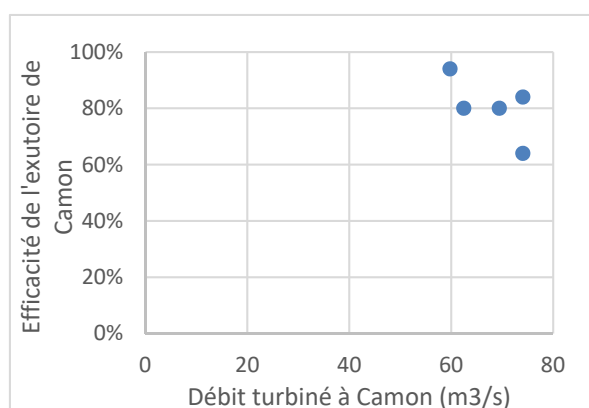
Figure 20 : Résultats d'efficacité de l'exutoire de Camon pour chaque lot de smolts marqués en fonction des débits turbinés à l'usine.
