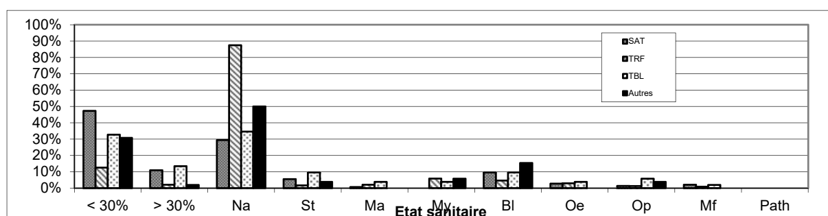
Figure 8 : Proportion de chacune des anomalies sanitaires relevées sur les individus classés « non sains » échantillonnés à Camon et à Pointis de Rivière en 2018
