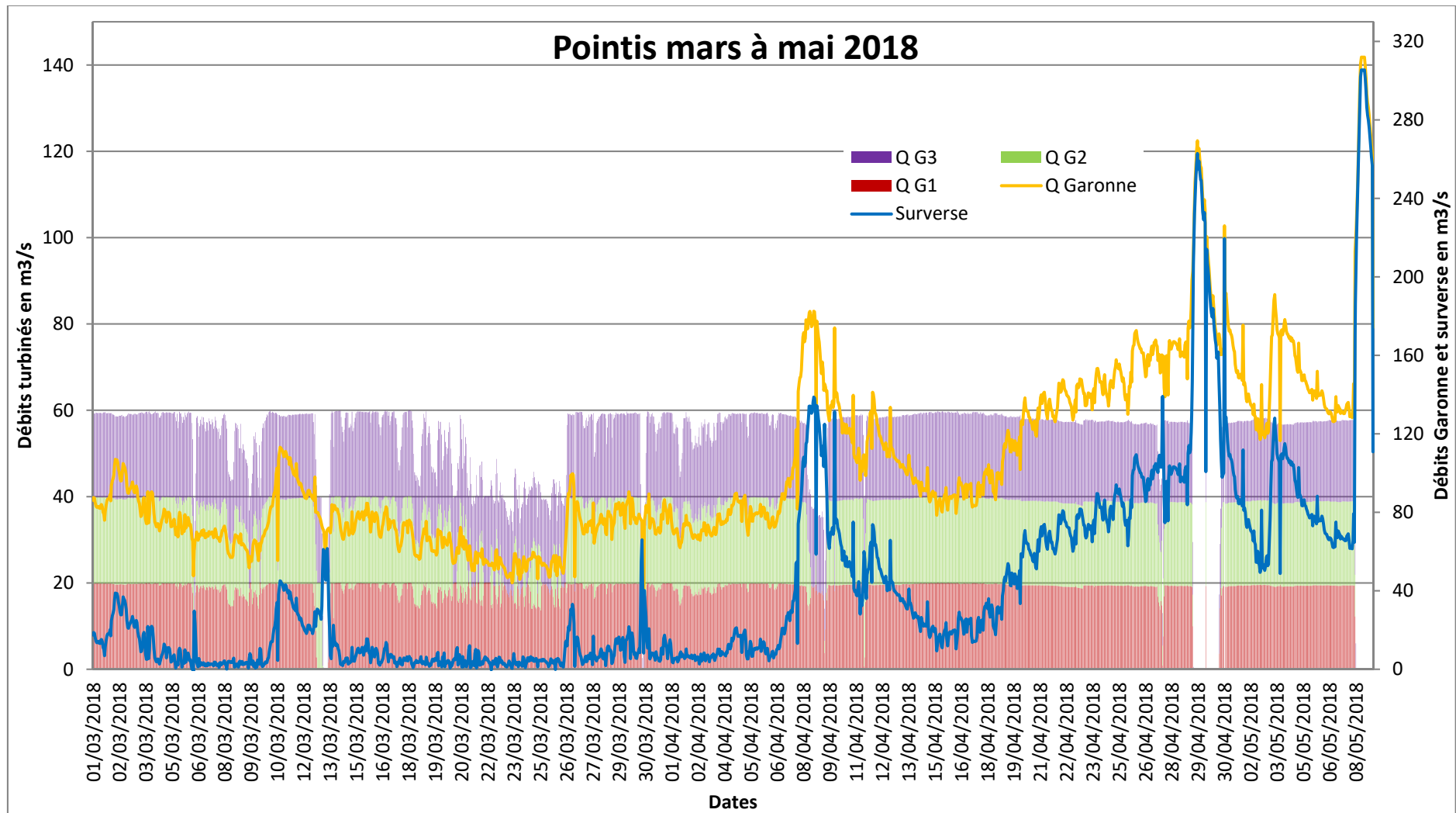
Figure 5 : Fonctionnement des groupes de l'usine de Pointis et débit de la Garonne durant la campagne 2018 (débit en m 3 /s)
