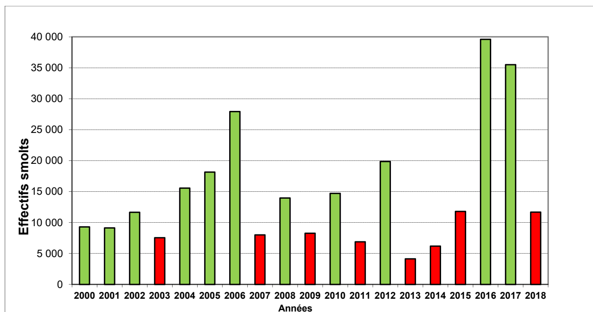
Figure 21 : Comparaison des effectifs de smolts de saumon capturés annuellement à Camon et Pointis (histogrammes rouges : années de forte hydrologie, histogrammes verts : années avec une hydrologie faible à moyenne).
