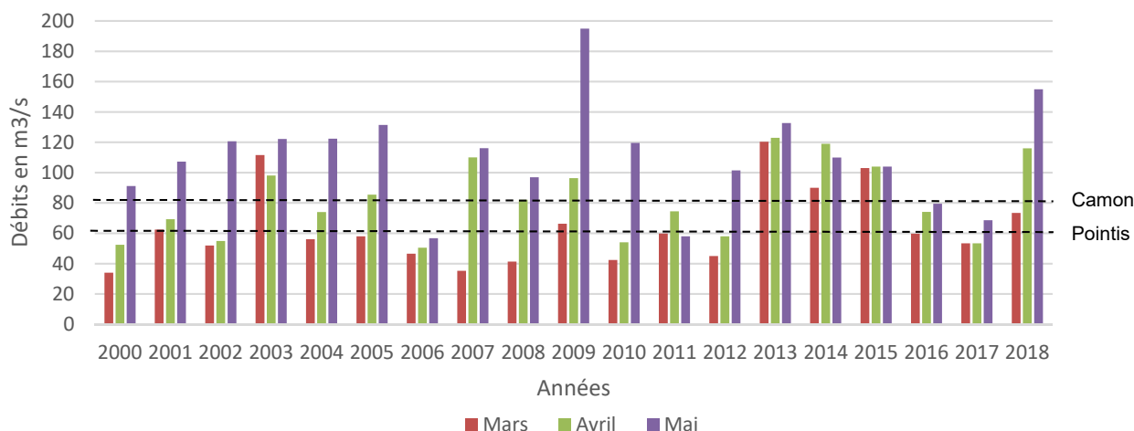
Figure 12 : Comparaison des débits journaliers de la Garonne mesurés à Valentine ou à Gourdan-Polignan de 2000 à 2018 (en pointillé niveau d'équipement des centrales)
