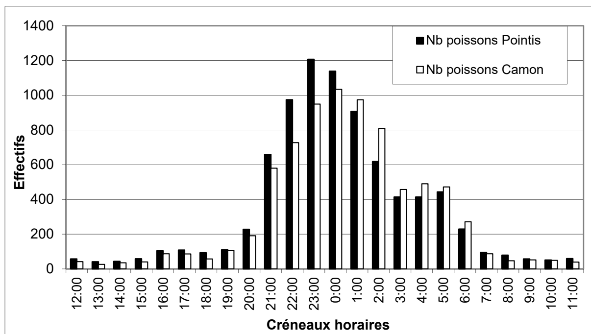
Figure 6 : Evolution des effectifs cumulés par créneaux horaires d'1 heure à Camon et à Pointis en 2018
